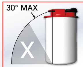
FIG. B: SENSOR TILT THRESHOLD FIG. B: LÍMITE DE INCLINACIÓN DEL SENSOR
