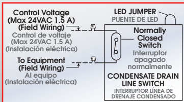
FIG. C: WIRING DIAGRAM FIG. C: DIAGRAMA ELÉCTRICO
