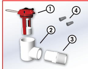
FIG. A: PRODUCT COMPONENTS FIG. A: COMPONENTES DEL PRODUCTO
