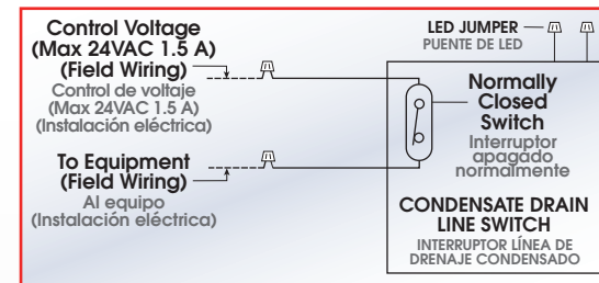
FIG. E: WIRING DIAGRAM WITH CUT JUMPER WIRE FIG. E: DIAGRAMA DE CABLEADO CON CORTE DEL CABLE DE PUENTE
